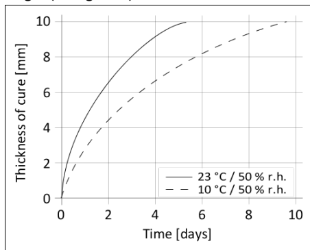
Figuur 1: Doorhardingsnelheid Sikaflex®-228
